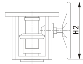
手轮装置
